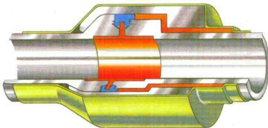
Рис.1 Конструкция электроизолирующей вставки (муфты)
