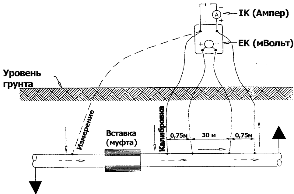
Рис.4 Схема коммутации контрольно-измерительного пункта при определении процента утечки через вставку (муфту).
